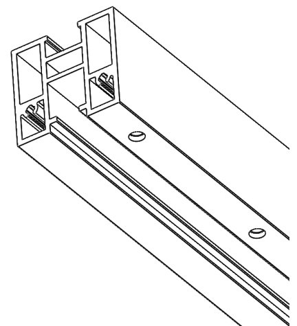
OJO Perfil inferior ya mecanizado Lower profile machined
