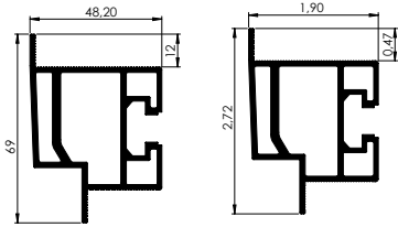
Perfil puerta Door profile
